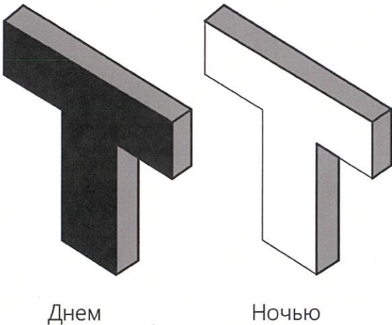
Вид ночью Вид днем Конструкция плоских вывесок с контурной подсветкой Подпись Дата г.Астана, район Сарайшык, улица Шамши Калдаяков, 1 Исполнитель Естаева Н.Б. 12.04 Конструкции вывесок Разработчик Зам.дир Ермекбай Д.А. КГУ "Астана-Жарнама" акимата г.Астаны Лист 4.2
