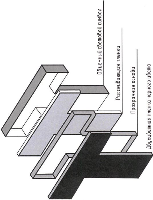
Конструкция
